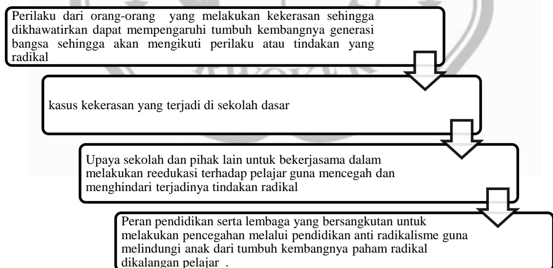
Gambar 2.2 Kerangka Piikir
