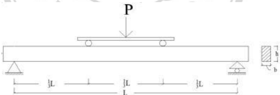
Gambar 2.3 Pengujian Kuat Lentur Balok (SNI 4431-2011)
