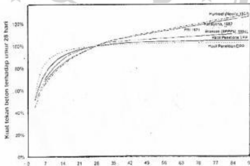
Gambar 2.4 Umur Beton (SNI 03-2834-2000)
