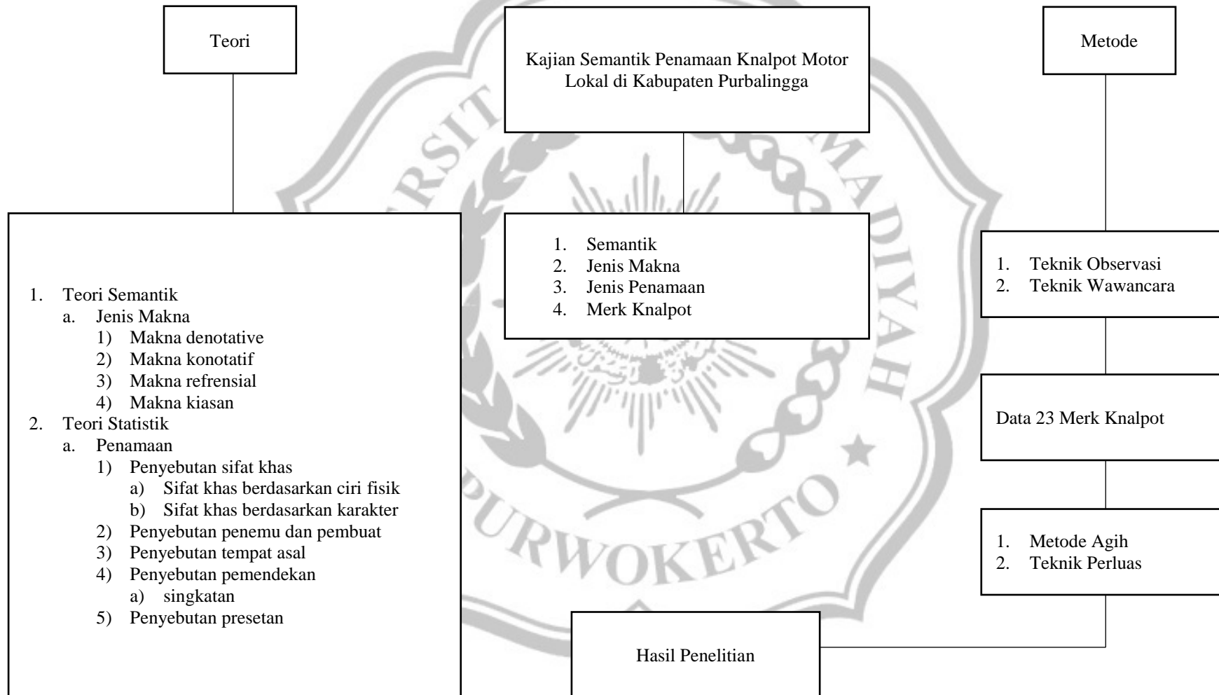
Gambar 2.1 Kerangka Teori
