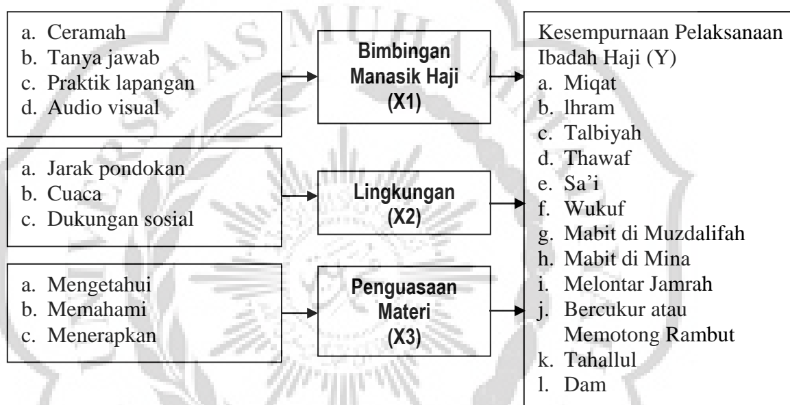
Gambar 2. 1. Kerangka Pikir
