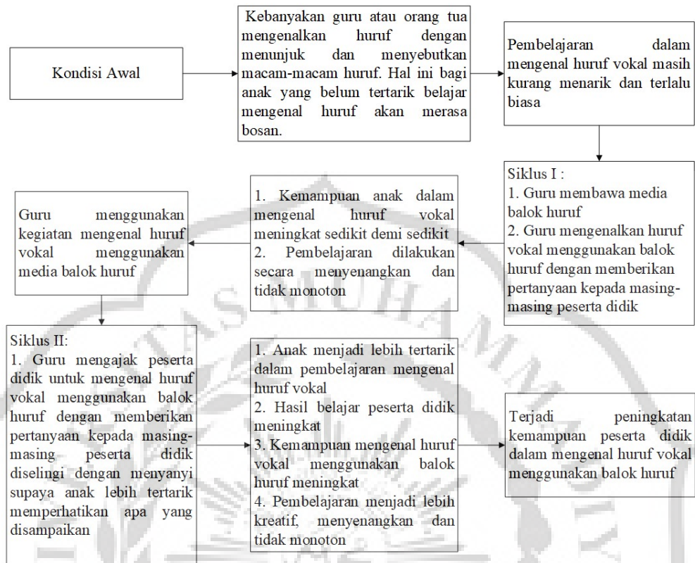
Gambar 2. 1 Kerangka Berpikir
