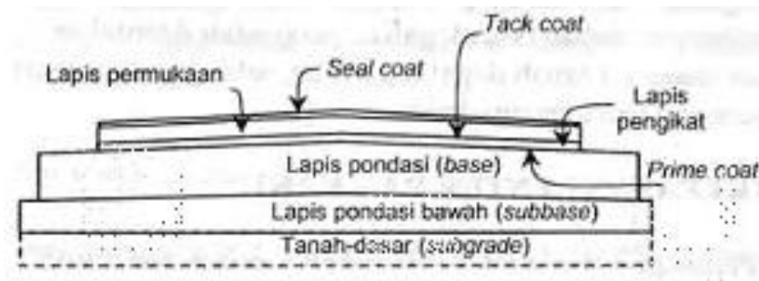
Gambar 2.4 Lapisan Konstruksi Perkerasan Lentur
