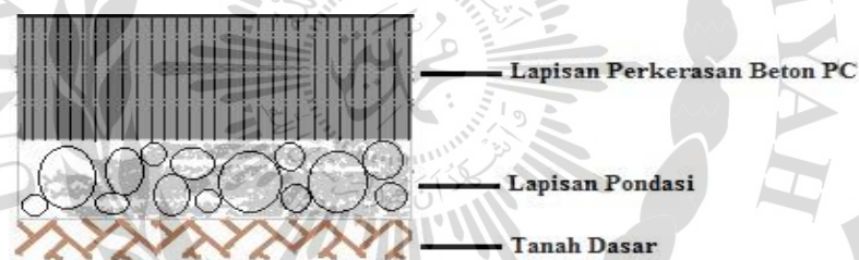
Gambar 2.2 Susunan lapis perkerasan rigid
