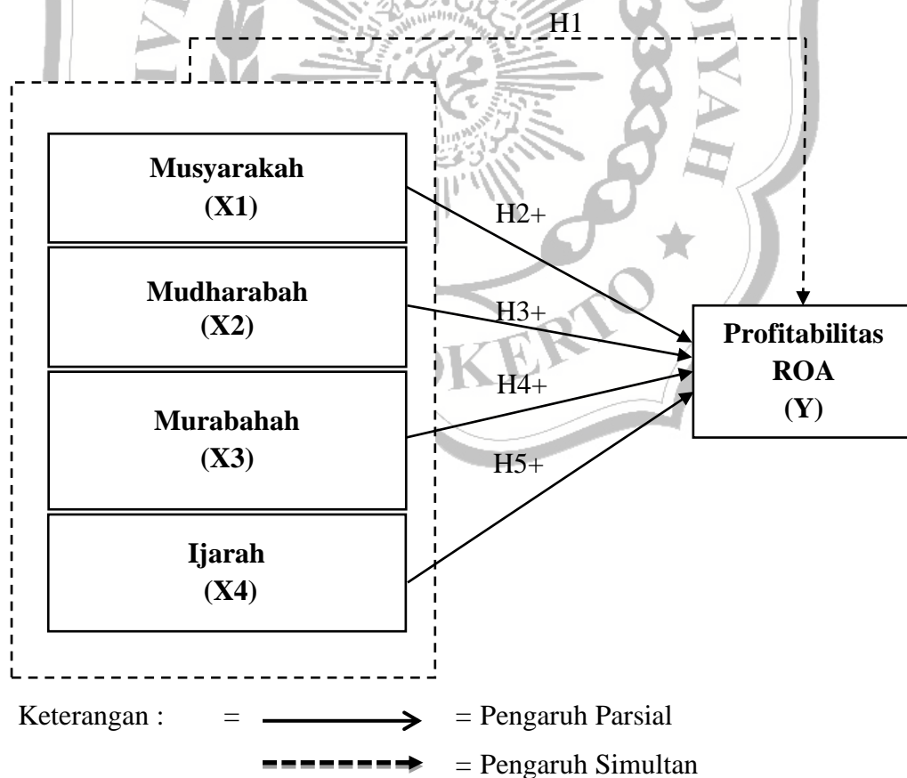
Gambar 2.1 Kerangka Pemikiran
